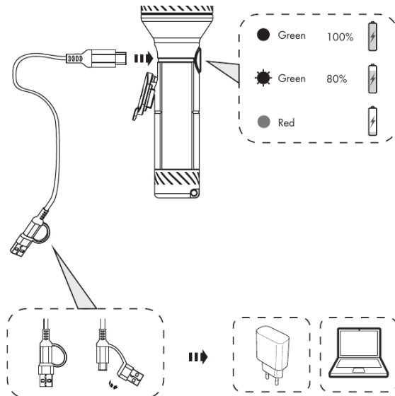
Laden in der Lampe per USB-Kabel – Stecker, Powerbank oder Laptop als Quelle.
